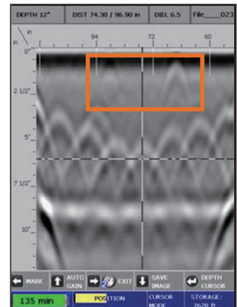
1,5cm 플라스틱 도관 측정 (철근 배근 위)
