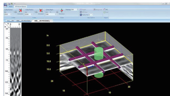
사용자가 지정한 가상 시추공 위치를 배경도 위에 입체적으로 표현.
